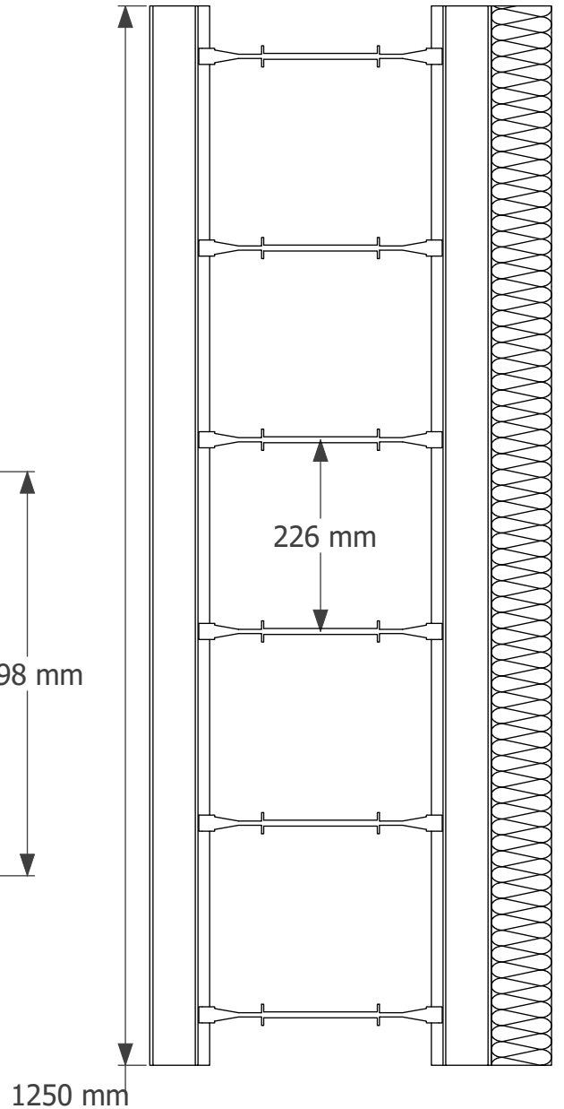
SCALE 1 : 8
