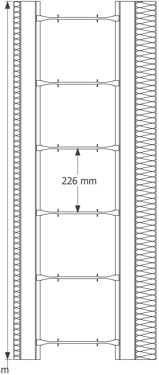
SCALE 1 : 8
