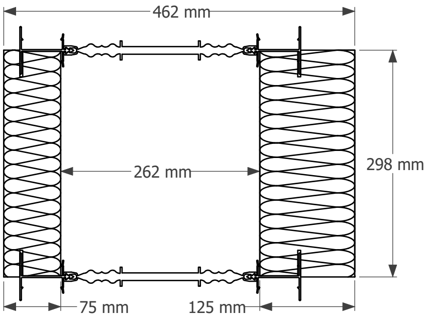
SCALE 1 : 5
